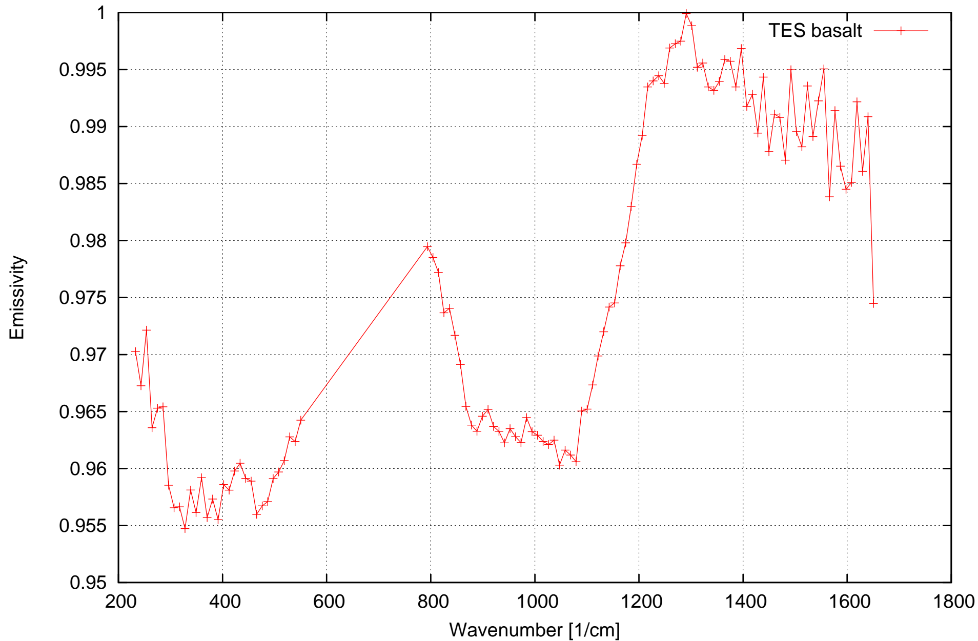
Mars basalt(TES)
